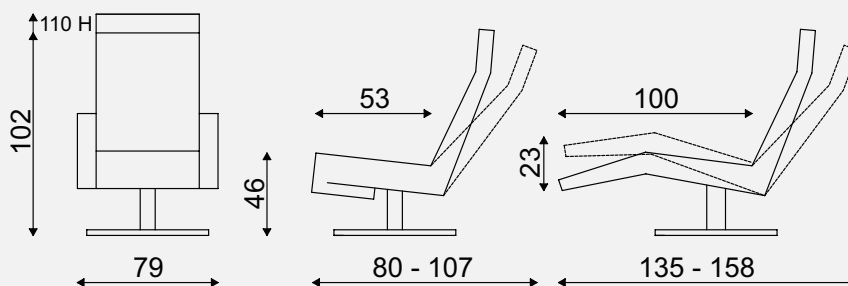
De getoonde afmetingen gelden voor de fauteuil in medium uitvoering
